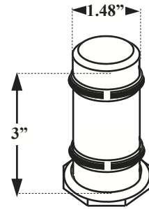
-14- GRIP RING STEM
