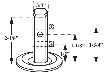
-41B- OCTAGON STEM
