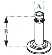
GRIP RING STEM
