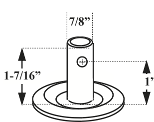
-31- ROUND STEM
