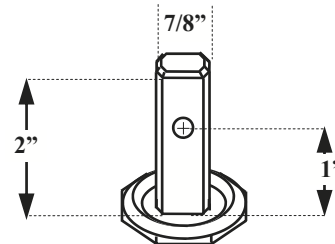
-42- OCTAGON STEM
