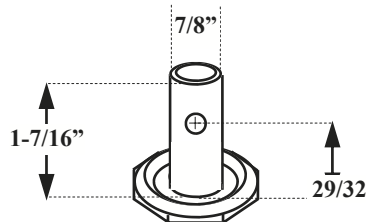
-31- ROUND STEM
