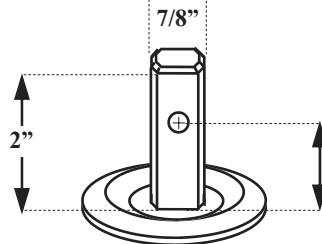
-42- OCTAGON STEM
